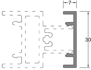
Çift Yön Açıklı Kayıt Ön Kapak Profili
