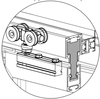
D : Taşıyıcı araba detayı
