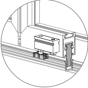
E : Kılavuz araba detayı
