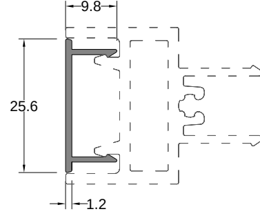
Kayıt Arka Kapak Profili
