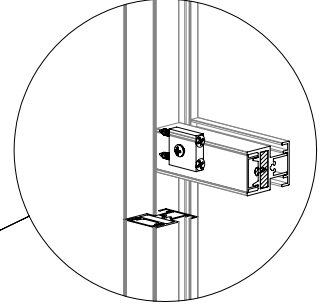
H : Karolaj detayı
