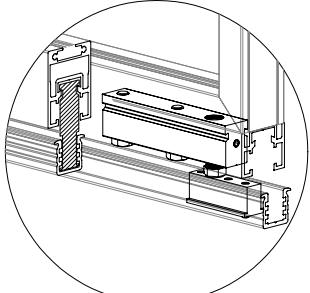
C : Alt pivot detayı
