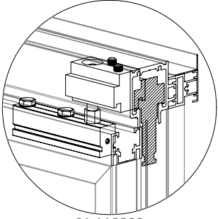
B : Üst pivot detayı
