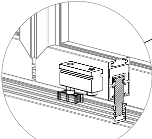
E : Kılavuz araba detayı
