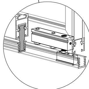
C : Alt pivot detayı
