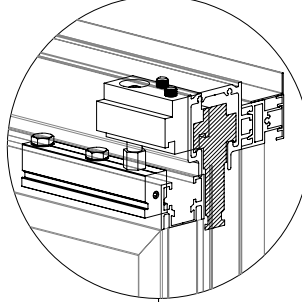
B : Üst pivot detayı
