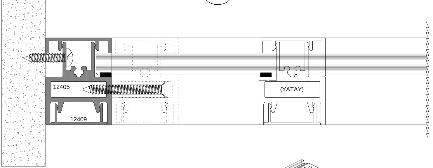
G : Üst ray/Yatay kayıt detayı
