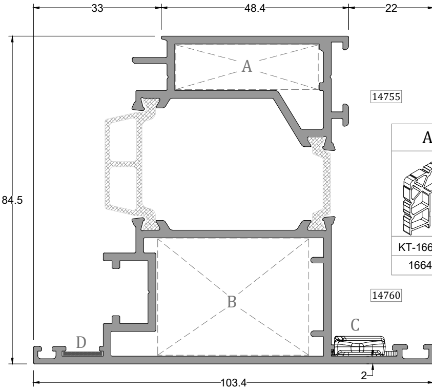
Dışa Açılır Pvc Kanallı Kanat Profili OUTWARD OPENING PVC GROOVE SASH PROFILE
