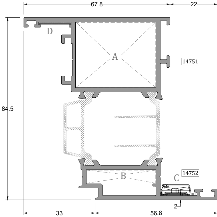
Euro Kanallı Kanat Profili EURO GROOVE SASH PROFILE
